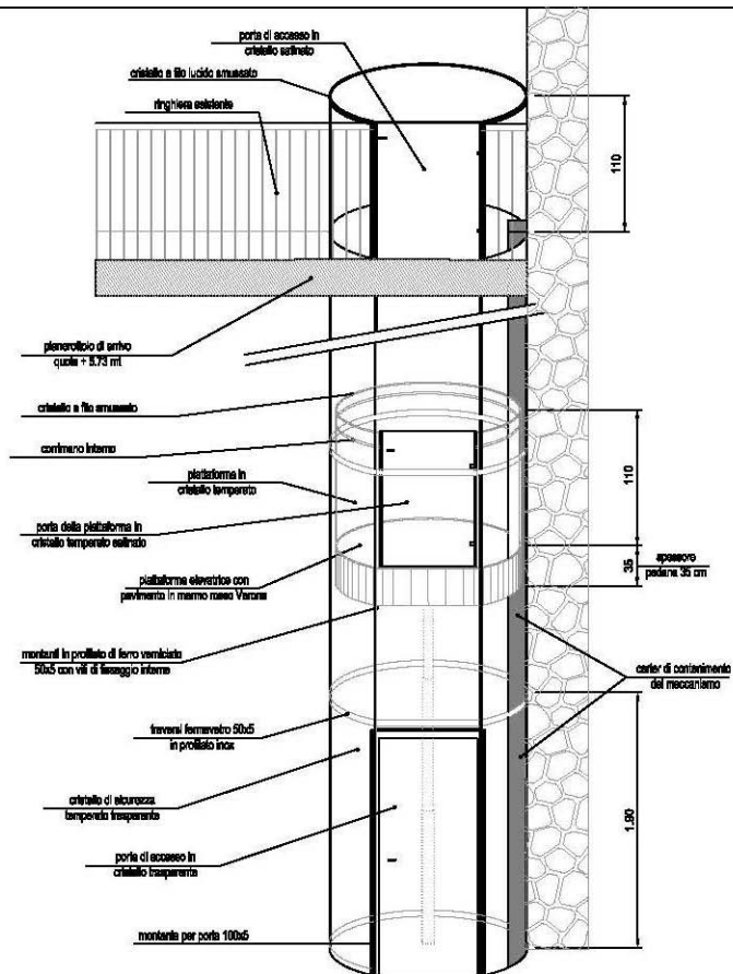
ASSONOMETRIA piattaforma elevatrice oleodinamica
